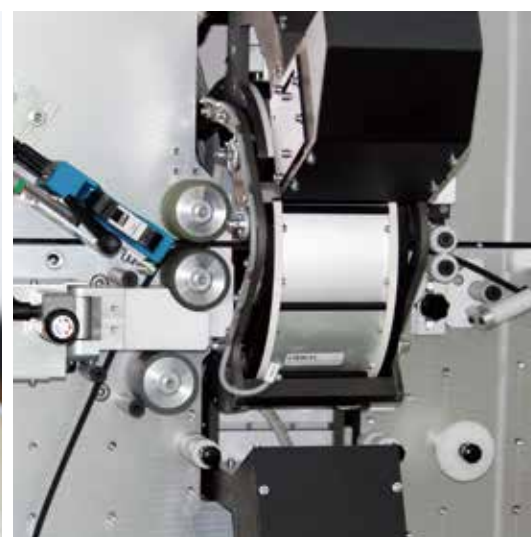
用于大尺寸O形圈的尺寸控制机
