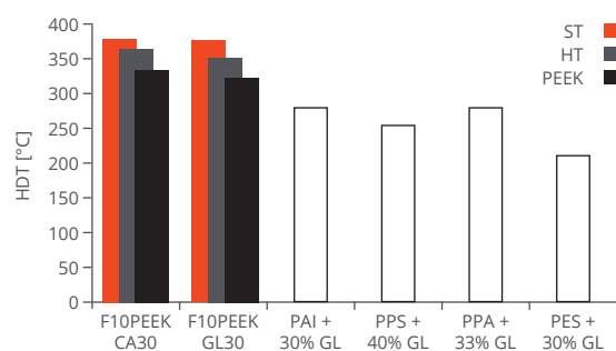
图6:F10PEEK材料和其他高性能聚合物的热变形温度(1.8 MPa)
