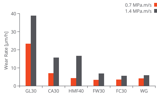
图10:使用止推垫圈方法测试的各种F10PEEK材料在低PV水平下的平均磨损率
