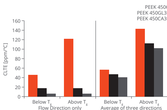
图7:低于和高于T g 的各种F10PEEK材料的线性热膨胀系数(CLTE)
